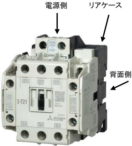
図 1: 製品外観(S-T21)
