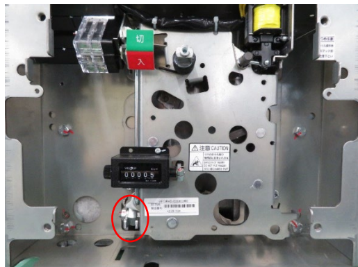
図1. VF-8D/13D 用操作機構(外観) (例)パネル固定[据付方式 P]形 手動ばね操作
