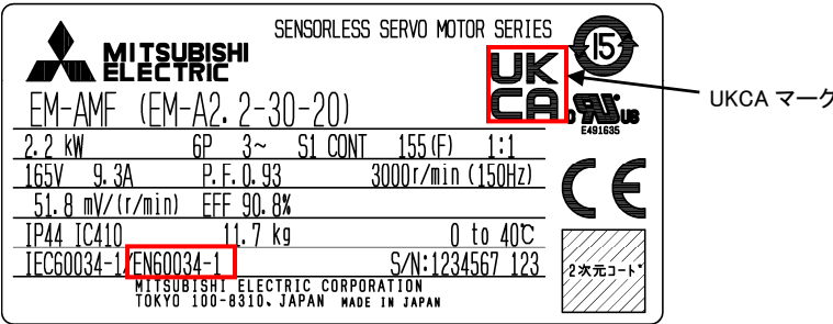
図1 定格銘板の例
