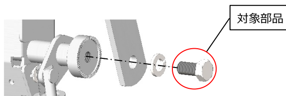
図 2. 操作ハンドル固定ボルト部構造
