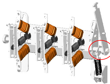
図 1. DV-3 形 外観及び変更箇所
